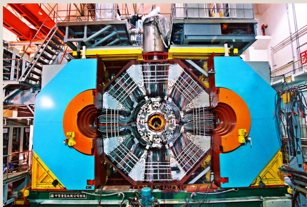
BES III探测器照片
