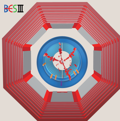
在BES III探测器上重建出的一个 J/\psi 粒子衰变过程的示意图
